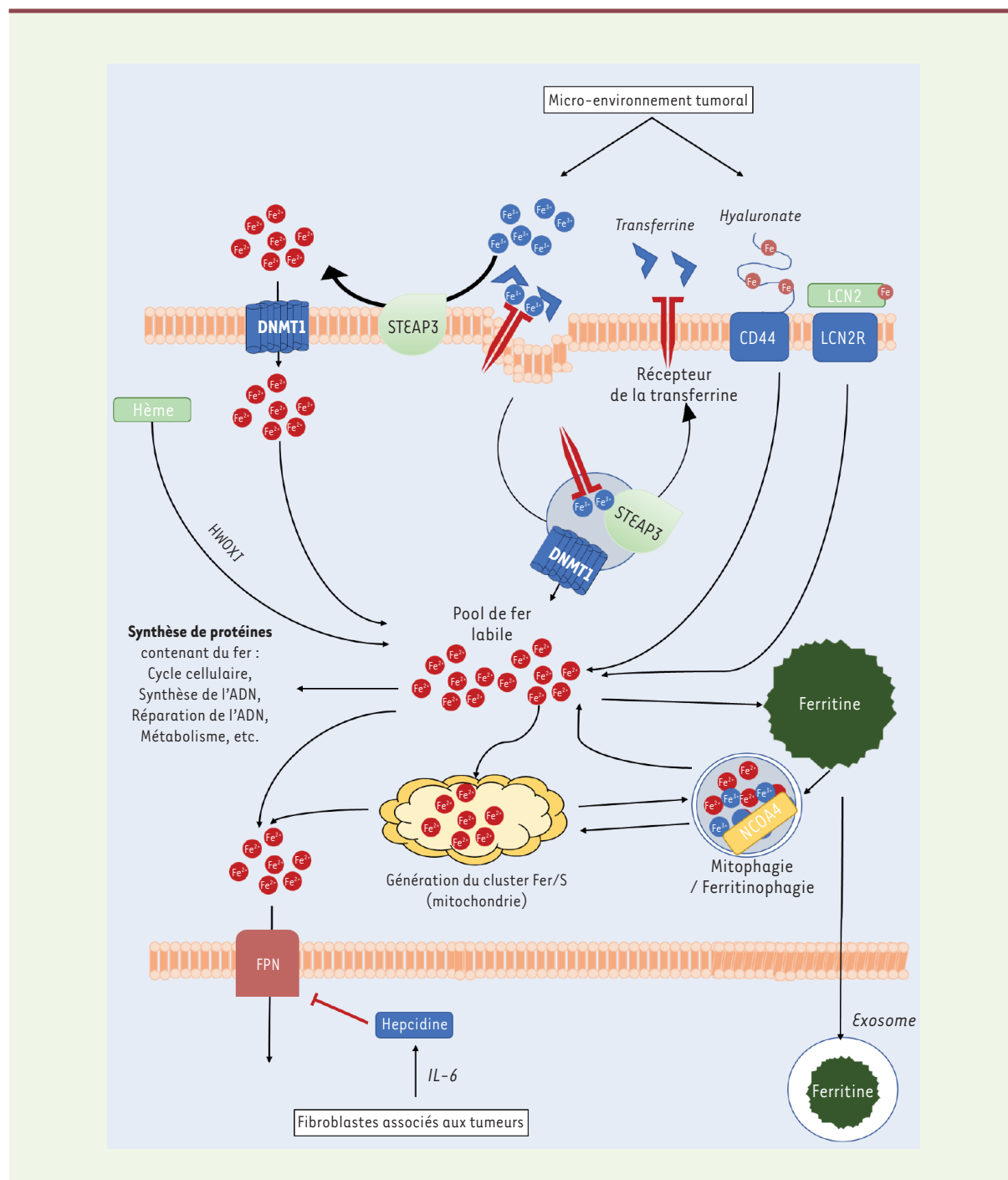
Figure 2. Métabolisme du fer intracellulaire. Fe^{3+} se lie à la transferrine (Tf) pour former le complexe Fe^{3+} -Tf, qui se lie au récepteur de la transferrine TfR1. L'ensemble est internalisé par endocytose. Dans l'endosome, l'acidification conduit à la libération du Fe^{3+} de la Tf, l'apo-Tf (la Tf dépourvue de fer) restant liée au TfR1. Le Fe^{3+} de l'endosome est réduit en Fe^{2+} par la ferriréductase STEAP3 ( six-transmembrane epithelial antigen of the prostate 3 ) et transporté dans le cytoplasme par DMT1 ( divalent metal transporter 1 ). Le complexe apoTf-TfR1 est recyclé à la membrane. Après son entrée dans le cytoplasme, le Fe^{2+} est conjugué avec des ligands du fer, formant le pool de fer labile cytosolique. Ce fer peut être stocké sous forme de ferritine, transféré à la mitochondrie, ou encore exporté de la cellule par la ferroportine 1. LCN2 : lipocaline 2 ; IL-6 : interleukine 6 ; FPN : ferroportine.
